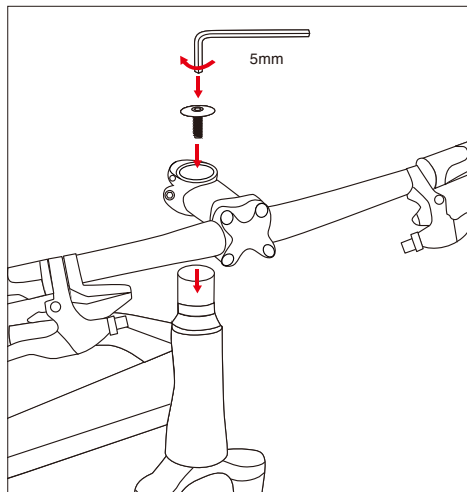
3. Instale el manillar y el vástago como se muestra en la imagen de arriba, asegurándose de que ninguno de los cables esté retorcido o demasiado apretado (es posible que tenga el manillar torcido). Coloque la tapa superior con el tornillo en el vástago y apriete el tornillo para asegurar el vástago hacia abajo en el tubo principal.
