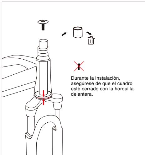
2. Retire la tapa superior y el tubo de plástico.
