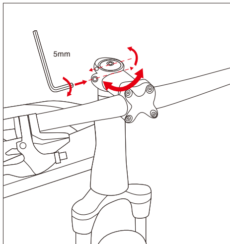
4. Alinee el manillar verticalmente con la rueda (es posible que deba aflojar el tornillo del paso 3 para hacer pequeños ajustes) y apriete los pernos en ambos lados del vástago.
