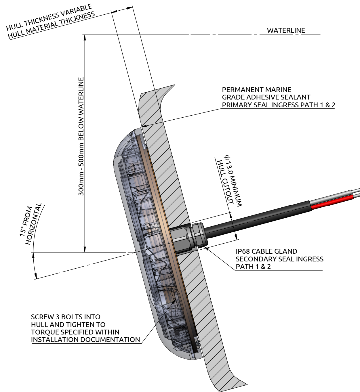
SECTION A-A
